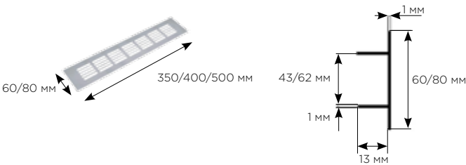
СХЕМА И РАЗМЕРЫ СИСТЕМЫ:
