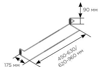
СХЕМА И РАЗМЕРЫ СИСТЕМЫ:
