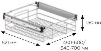
СХЕМА И РАЗМЕРЫ СИСТЕМЫ:
