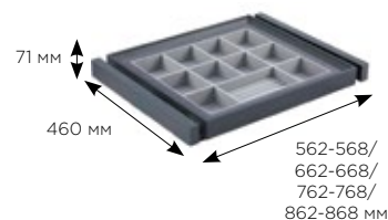
СХЕМА И РАЗМЕРЫ СИСТЕМЫ:
