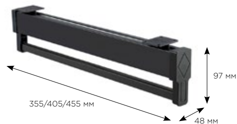
СХЕМА И РАЗМЕРЫ СИСТЕМЫ:
