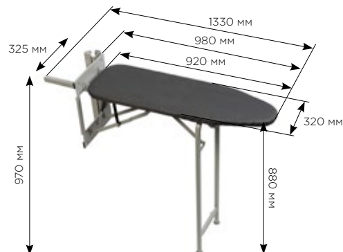
СХЕМА И РАЗМЕРЫ СИСТЕМЫ И КОРПУСА:
