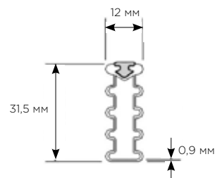
Комплект держателей с заглушками Арт. 18200086
