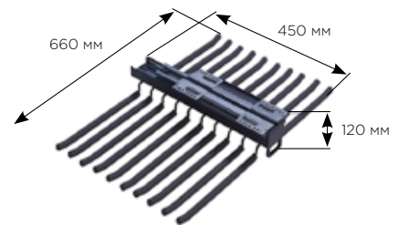
СХЕМА И РАЗМЕРЫ СИСТЕМЫ:
