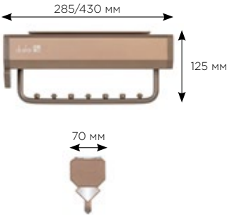
СХЕМА И РАЗМЕРЫ СИСТЕМЫ:
