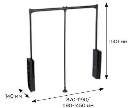
СХЕМА И РАЗМЕРЫ СИСТЕМЫ:
