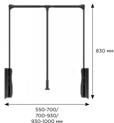
СХЕМА И РАЗМЕРЫ СИСТЕМЫ:
