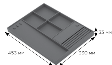
СХЕМА И РАЗМЕРЫ СИСТЕМЫ:
