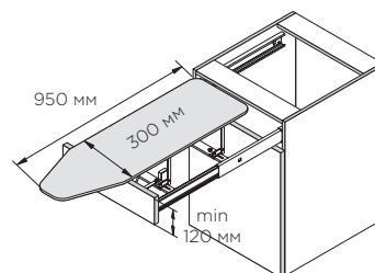
СХЕМА И РАЗМЕРЫ КОРПУСА:
