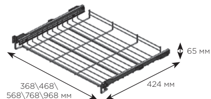
СХЕМА И РАЗМЕРЫ СИСТЕМЫ:
