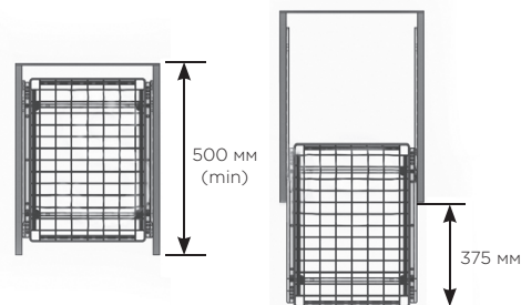
СХЕМА И РАЗМЕРЫ КОРПУСА:
