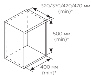
СХЕМА И РАЗМЕРЫ КОРПУСА:
