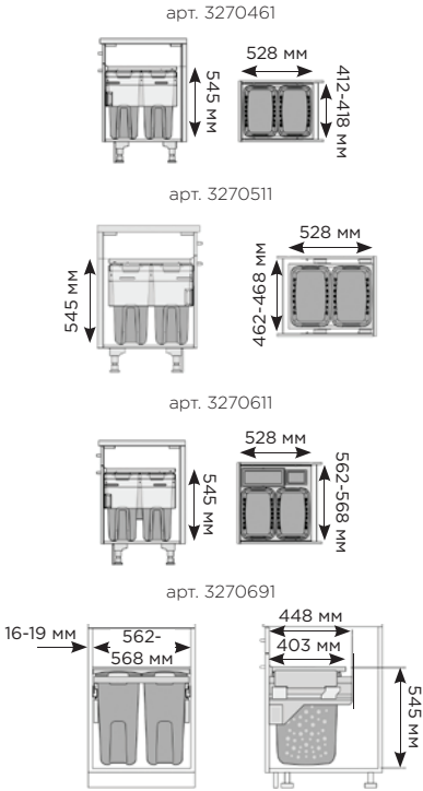
СХЕМА И РАЗМЕРЫ СИСТЕМЫ:
