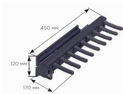
СХЕМА И РАЗМЕРЫ СИСТЕМЫ:
