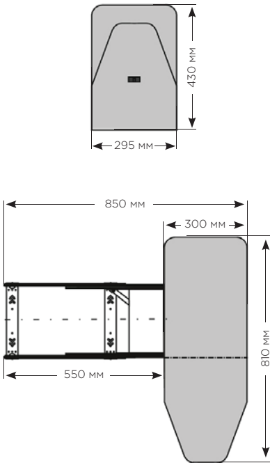
СХЕМА И РАЗМЕРЫ СИСТЕМЫ:
