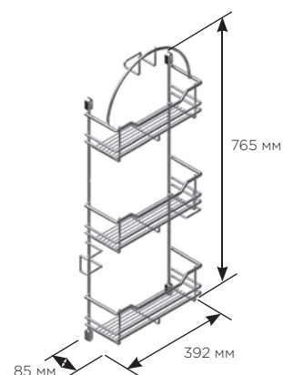
СХЕМА И РАЗМЕРЫ СИСТЕМЫ:
