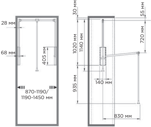
СХЕМА И РАЗМЕРЫ СИСТЕМЫ:
