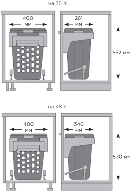
СХЕМА И РАЗМЕРЫ СИСТЕМЫ:
