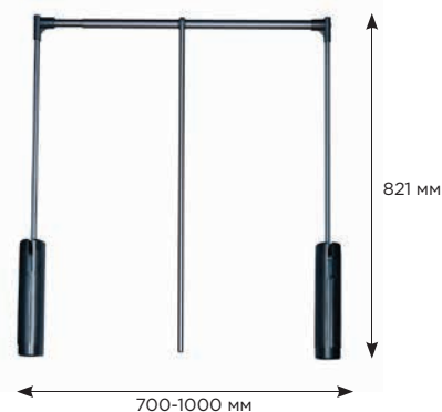
СХЕМА И РАЗМЕРЫ СИСТЕМЫ:
