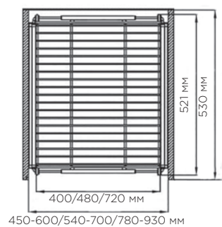
СХЕМА И РАЗМЕРЫ СИСТЕМЫ:
