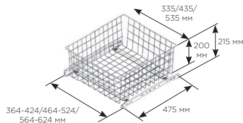
СХЕМА И РАЗМЕРЫ КОРПУСА:
