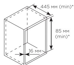
СХЕМА И РАЗМЕРЫ КОРПУСА:
